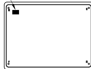
No. 3 数量标签 贴标签于真空盒左上角
