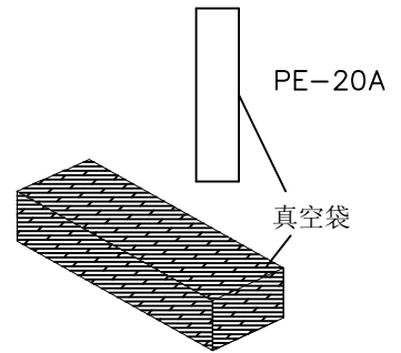
No: 4 将4扎包扎好的真空管装入真空袋, 外加2包干燥剂,机台抽真空 PE-20A规格: 35*95cm
