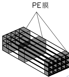
No: 3 20管为一扎 用PE膜固定每扎真空管两端及中间, 包住两端利角,以防划破胶袋
