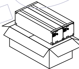
No: 6 内箱放入外箱(2内箱/外箱) 外箱规格: CTN-10C(双坑K=K 65*33*17CM)
