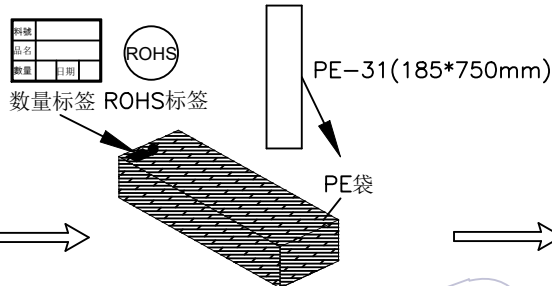
No: 3 20管为一扎套PE-31袋, 内附1包干燥剂 封口机封口, 封箱胶缠绕PE袋两端 再贴标签
