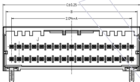
34P Y-KEY
